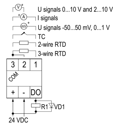
Fig. 6 Wiring diagram
