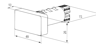
Fig. 3 Dimensions
